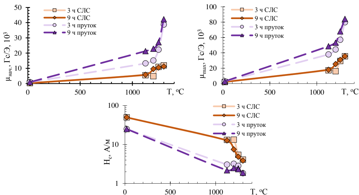
Рисунок 5 – Изменение магнитной проницаемости и коэрцитивной силы образцов из сплава 80НХС в зависимости от режима ТО
