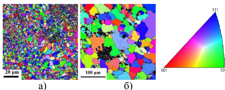
Рисунок 8 – EBSD анализ аддитивного – а) и литого – б) образцов сплава 25X15КА
