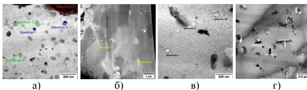
Рисунок 9 – Частицы различной морфологии и размеров в структуре аддитивного – а, б) и литого – в, г) образцов сплава 25X15КА
