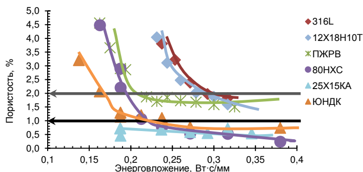
Рисунок 3 – Зависимость значений пористости от энерговложения
