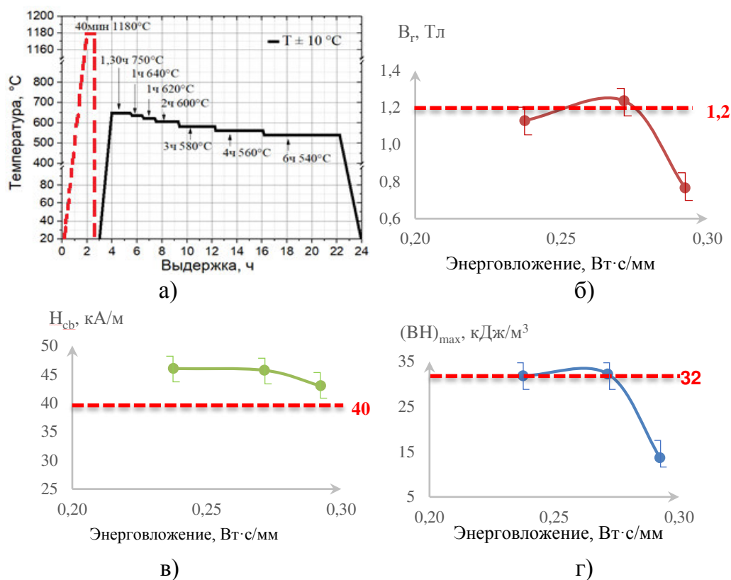
Рисунок 7 – Уточненный режим ТМО сплава 25X15КА – а) и усредненные магнитные свойства СЛС образцов из сплава 25X15КА в зависимости от энергозложения – б, в, г). Пунктирной линией показаны требования ГОСТ
