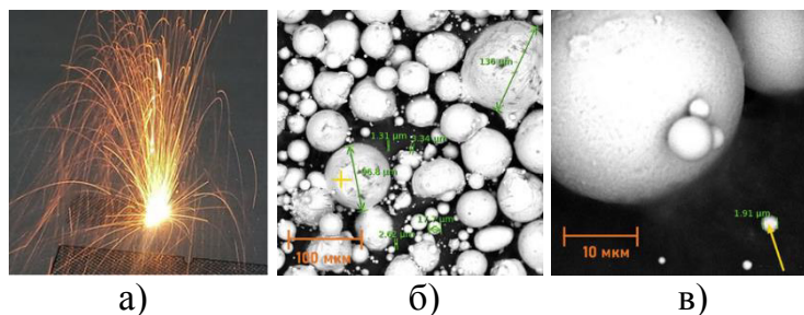
Рисунок 11 – Разлет частиц из зоны воздействия лазера – а) и СЭМ изображения “гари” 25X15К – б, в)
