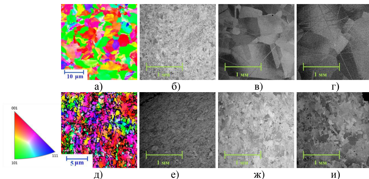
Рисунок 6 – EBSD анализ ковального – а) и СЛС – д) сплава 80НХС в исходном состоянии, а также микроструктура выточенных – б, в, г) и СЛС – е, ж, и) образцов: без ТО – б, е), ТО 1125^\circ\text{C} в течение 3 ч – в, ж), ТО 1300^\circ\text{C} в течение 9 ч – г, и)
